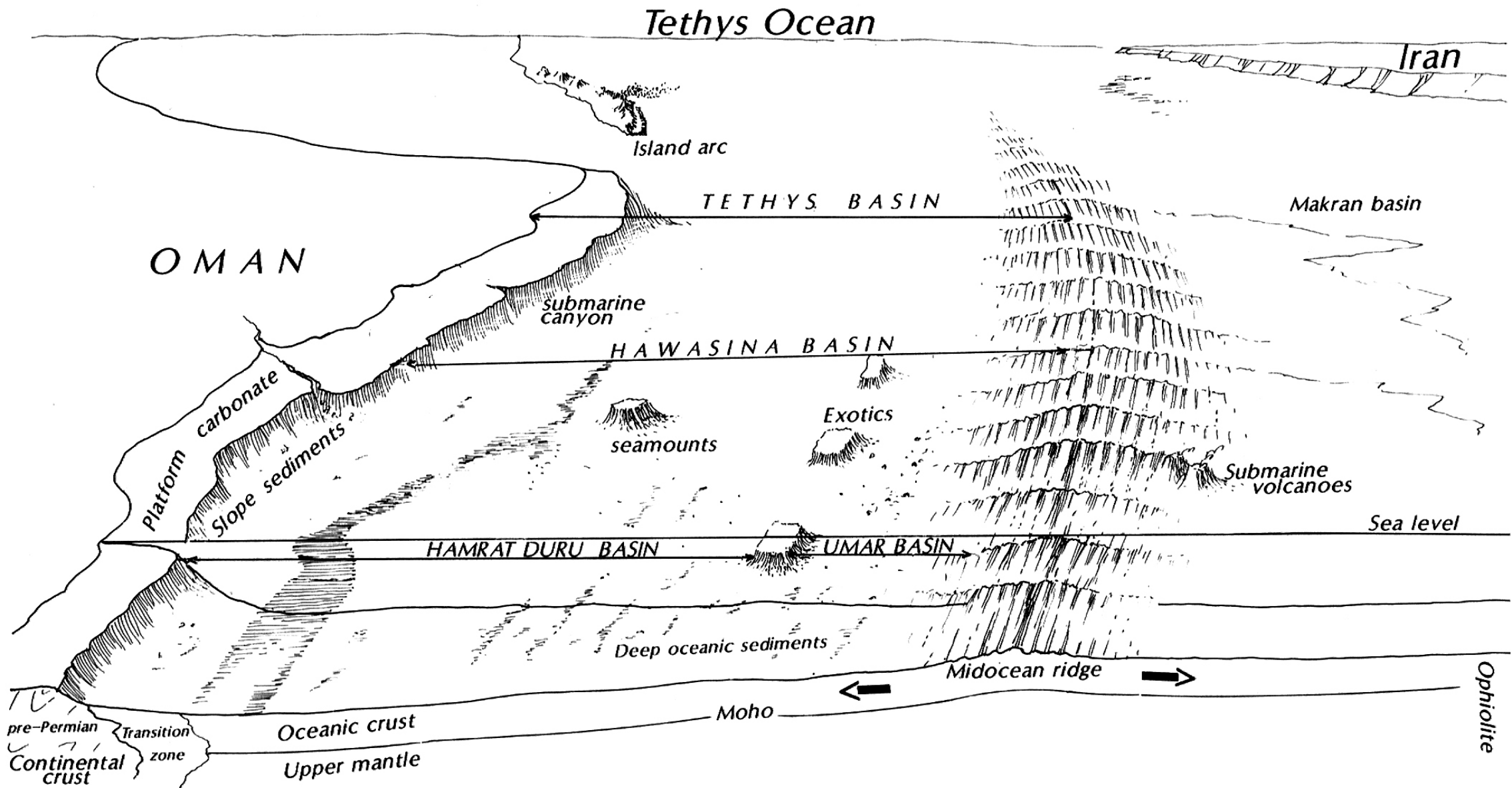
GÉOMÉTRIE DE LA MARGE OMANAISE
