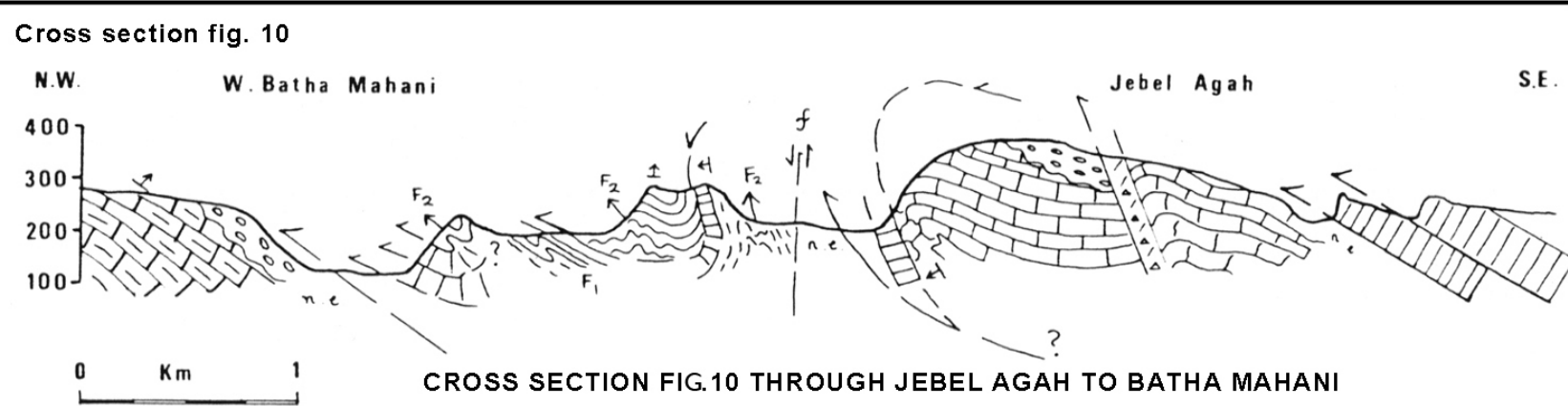
MARQUEURS TECTONIQUES DE LA RÉGION DU JEBEL QAMAR, DU JEBEL AGAH ET DU WADI BATHI MAHANI
