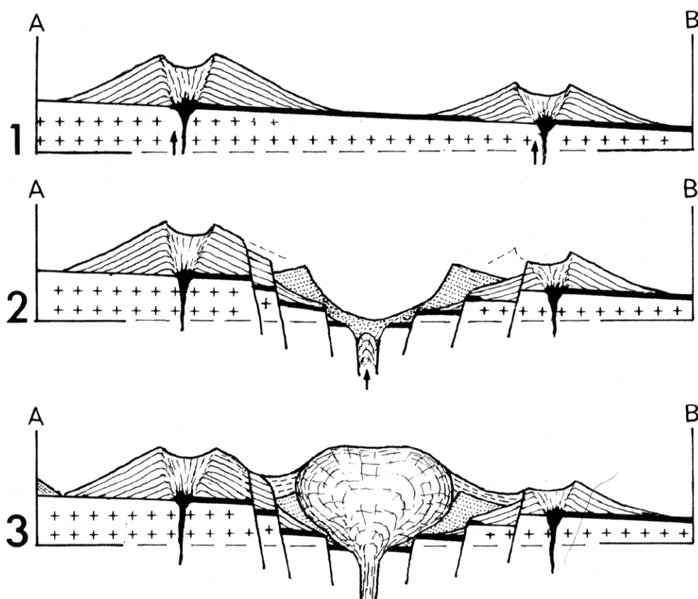
Système volcanique du Sarcouy 3 - coupe interprétative A-B au stade actuel 2-1 - étapes antérieures
